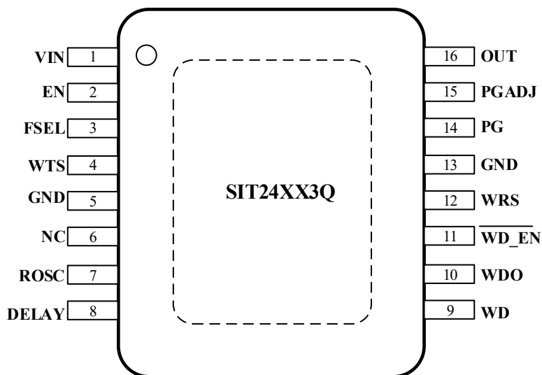
图 1 SIT24XX3Q 系列引脚分布图
