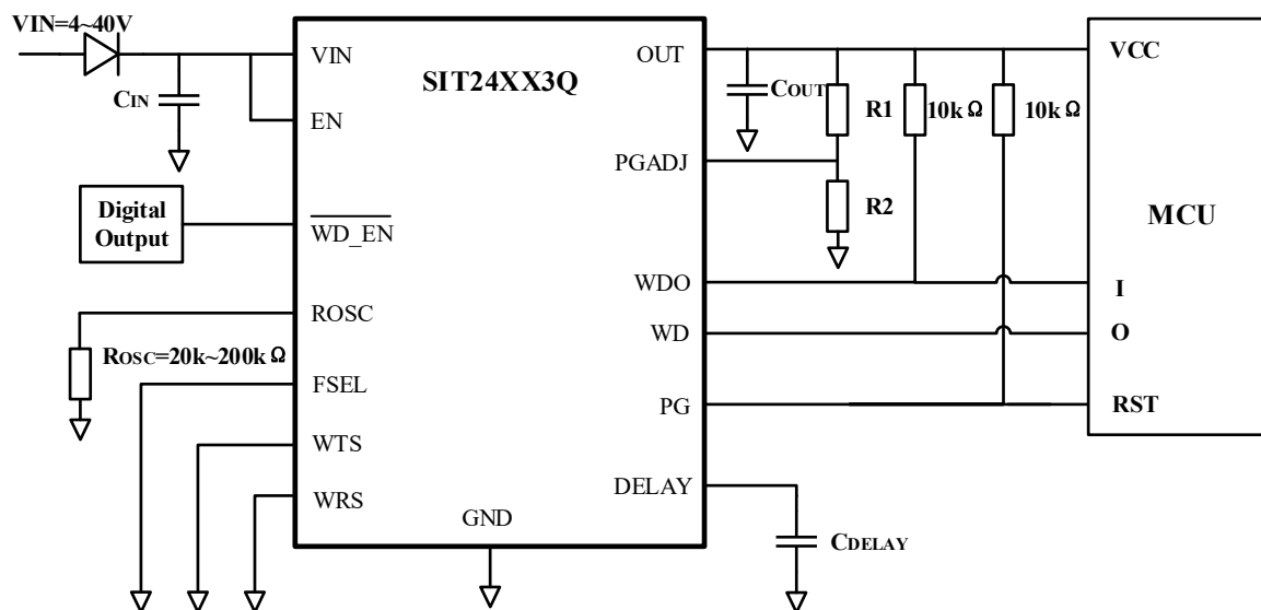
图 3 SIT24XX3Q 系列典型应用图
