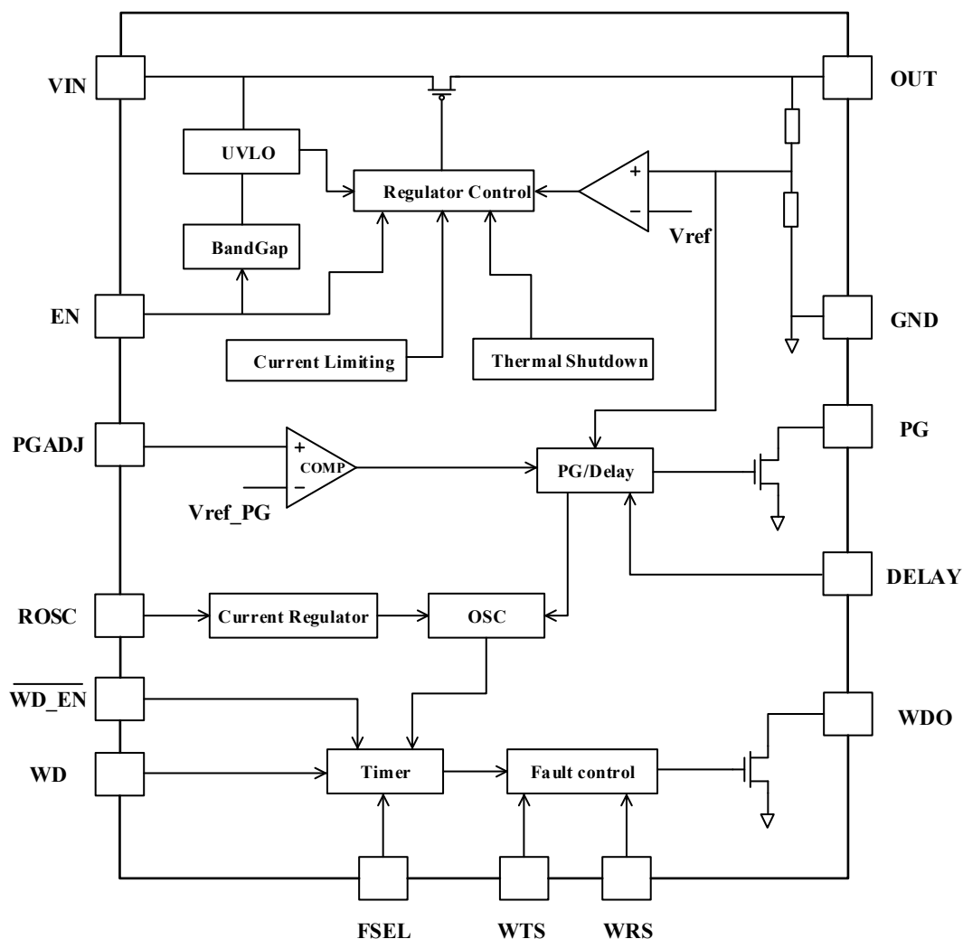
图 2 SIT24XX3Q 系列内部框图
